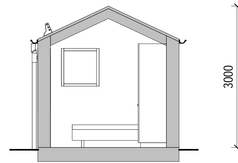
SEKTION A-A
